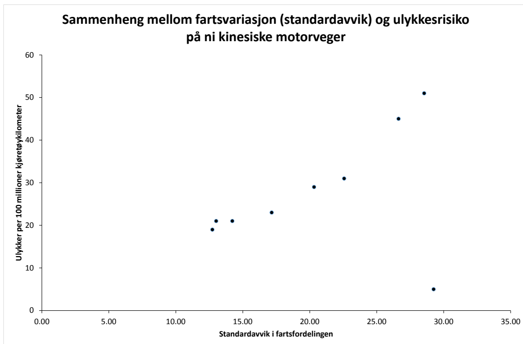
Figur 5.5: Sammenheng mellom standardavvik i fartsfordeling og ulykkesrisiko på ni motorveger i Kina. Kilde: Hou et al. 2010.
