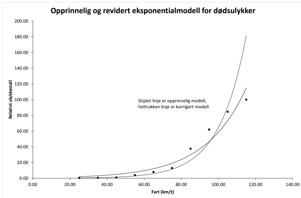
Figur 4.4: Opprinnelig og korrigert eksponentialmodell for dødsulykker.
