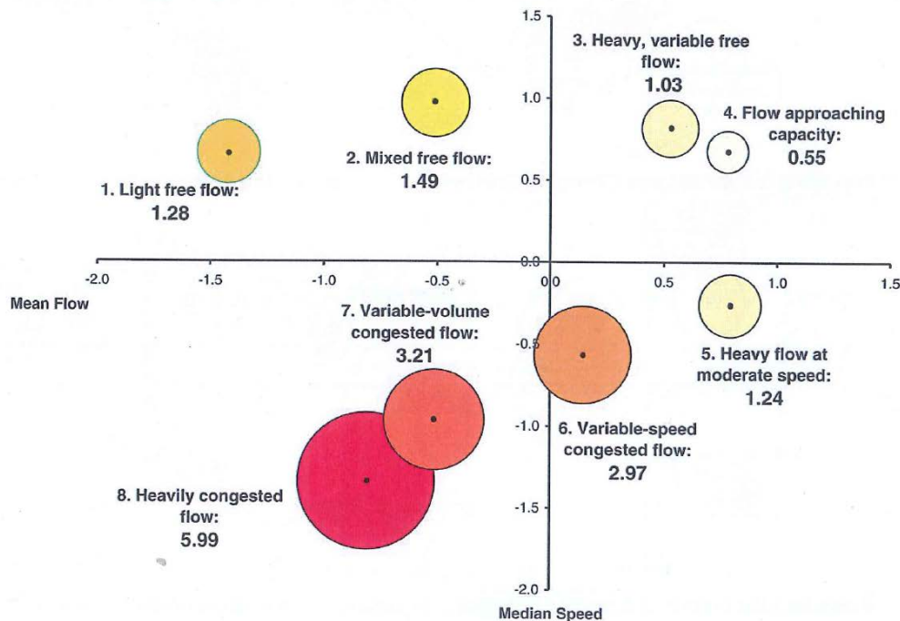
Figur 5.11: Ulykkesrisiko ved ulike trafikketilstander. Kilde: Golob et al. 2004.
