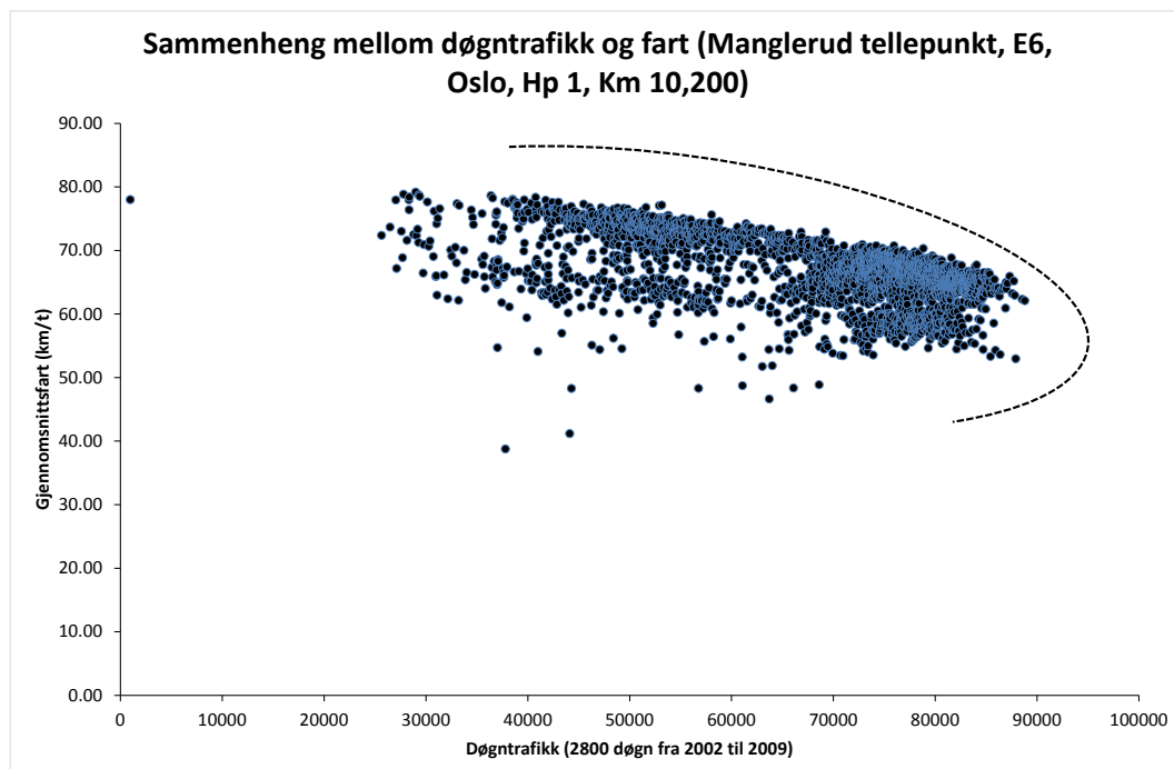
Figur 5.8: Sammenhengen mellom døgntrafikk og gjennomsnittsfart over døgnet i 2800 døgn ved Manglerud tellepunkt på E6 i Oslo.
