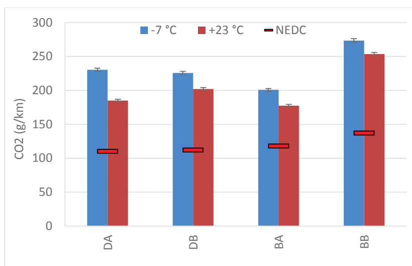
Figur 10: CO 2 -utslipp i g/km for to senest testede Euro 6 diesel-personbiler (DA og DB) og for to tilsvarende bilmodeller med bensinmotor (BA og BB). Den røde markeringen viser typegodkjenningensverdier som oppgitt av produsentene.
