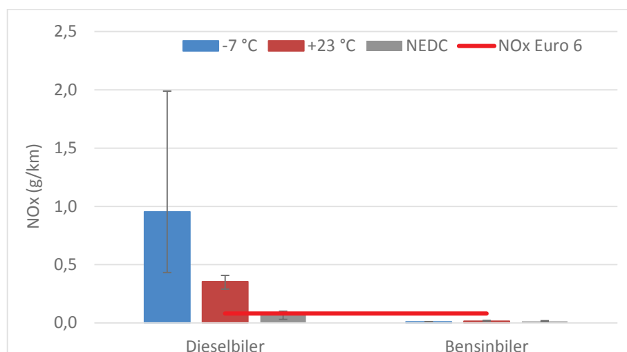
Figur 6: Gjennomsnitt NO x -utslipp i g/km, målt ved -7 og +23 °C for syv Euro 6 dieselbiler og tre Euro 6 bensinbiler ved kjøring av Helsinki bykjøringsyklus. Den grå søylen viser gjennomsnittet av typegodkjenningssyklusverdiene som oppgitt av leverandørene. I figuren vises også spredningen av målte verdier mellom de forskjellige bilene. Den røde linjen viser typegodkjenningskravet for Euro 6 diesel- og bensinbiler (0,08 g/km resp. 0,06 g/km).
