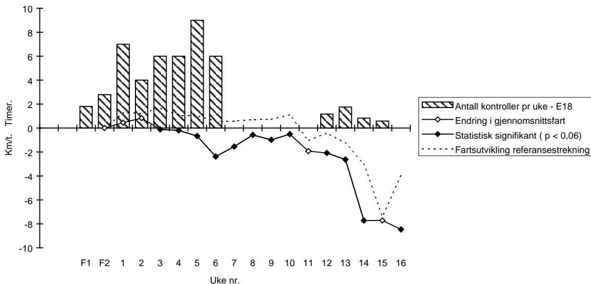
Figur 17. Endring i gjennomsnittsfart - E18 - Rogaland - kl 15-19. Nivå: 3 timer pr døgn.
