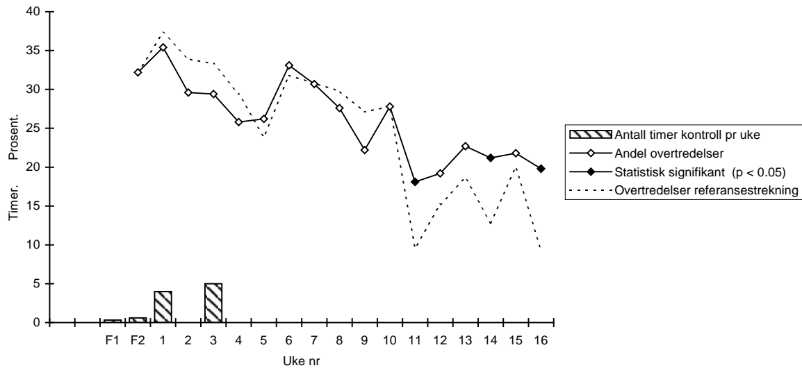
Figur 2. Endring i andel overtredelser (> 10 km/t over fartsgrensen). Riksvei 35/280 - Buskerud - kl 00-06. Nivå: 3 timer pr 3.døgn.
