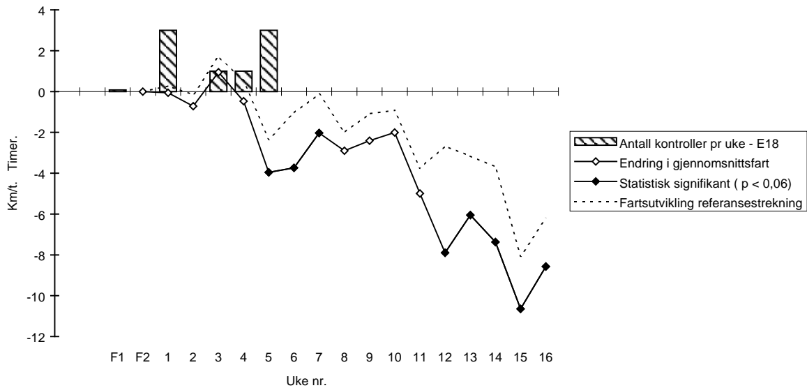
Figur 13. Endring i gjennomsnittsfart - E18 - Rogaland - kl 06-09. Nivå: 3 timer pr døgn.
