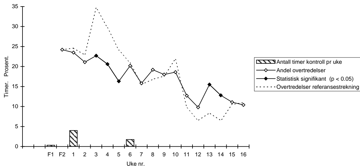
Figur 24. Endring i andel overtredelser (> 90 km/t). Fartsgrense: 80 km/t. Riksvei 2 - Akershus - kl 0609. Nivå: 4 timer pr døgn.
