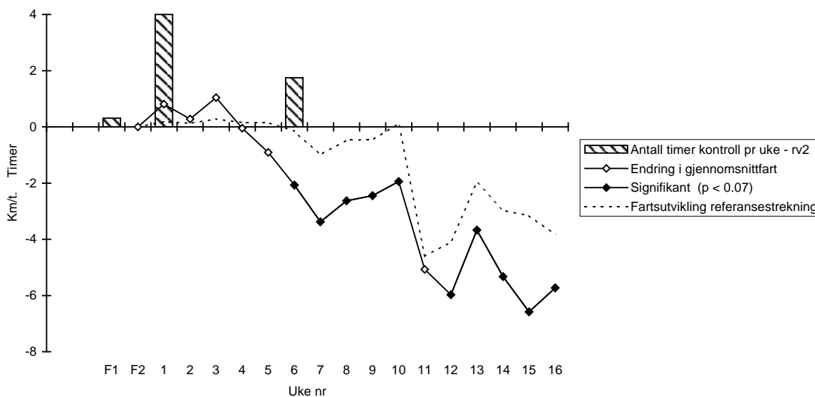
Figur 33. Endring i gjennomsnittsfart - riksvei 2 - Akershus kl 06-09. Sone: 60 km/t. Nivå: 4 timer pr døgn.
